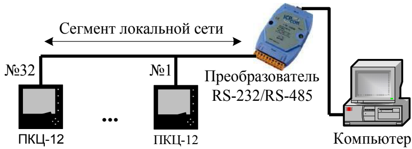
Рисунок 9 - Подключение через RS-485
